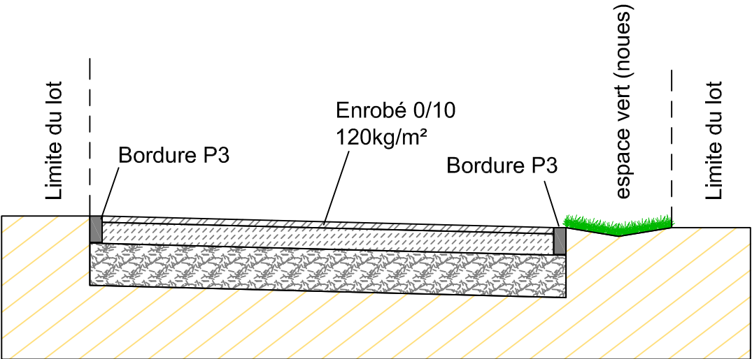
Profil en travers - coupe AA'
